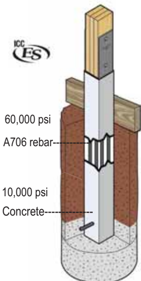
Precast Perma-Column®
